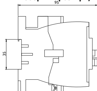
Габаритні розміри, mm
