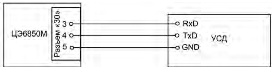
Рисунок 4.6 – Схема подключения интерфейсных линий EIA232
