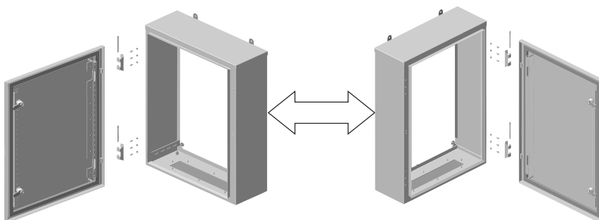
Предусмотрена возможность навески двери на разные стороны
