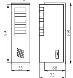
ROLO JQ-L
