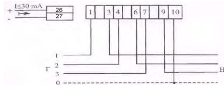
Рисунок 2 - Схема підключення лічильника ЦЭ6804-U у корпусі P31
