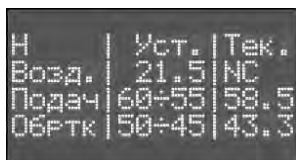
Рисунок 14.32 – Раздел Экран 1, датчик температуры воздуха заблокирован
