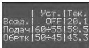
Рисунок 14.31 – Раздел Экран 1, нагрев выключен пользователем или таймером
