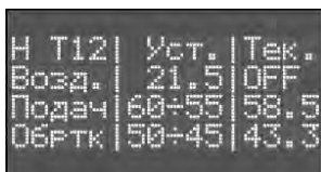
Рисунок 14.32 – Раздел Экран 1, датчик температуры воздуха заблокирован
