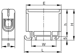
Рисунок 1 – KBC 6-50 (1/2, 1/3)
