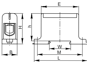
Рисунок 2 – KBC 16-95 (1/2), KBC 35-150
