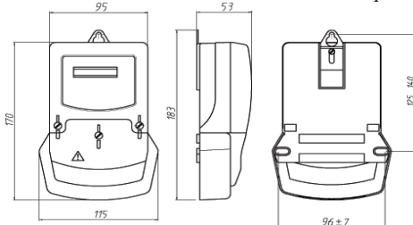
Рисунок 1 – Загальний вигляд лічильника ЦЭ6807Б-У в корпусі ШБ
