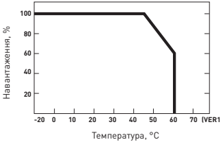
Рис. 2 – Перевантажувальна характеристика
