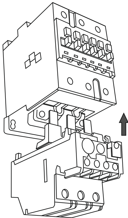
Можливість підключення теплого реле до магнітного пускача FC4
