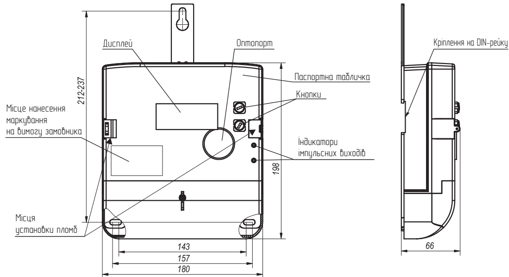
Малюнок А.1 - Загальний вигляд, габаритні і установчі розміри, місця установки пломб на корпусі трифазного лічильника прямого включення типу МТХ 3...0.D...4...3...4
