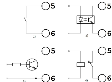
Мал. 2. Варіанти схем зовнішнього керування.
