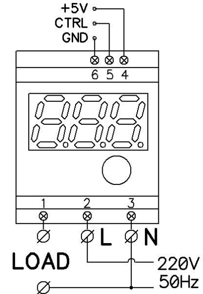
Мал. 1. Схема електричних з'єднань.
