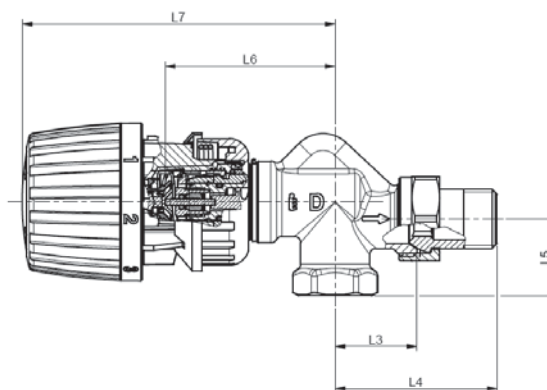
Осьовий клапан RA-DV з термостатичним елементом RA 2991
