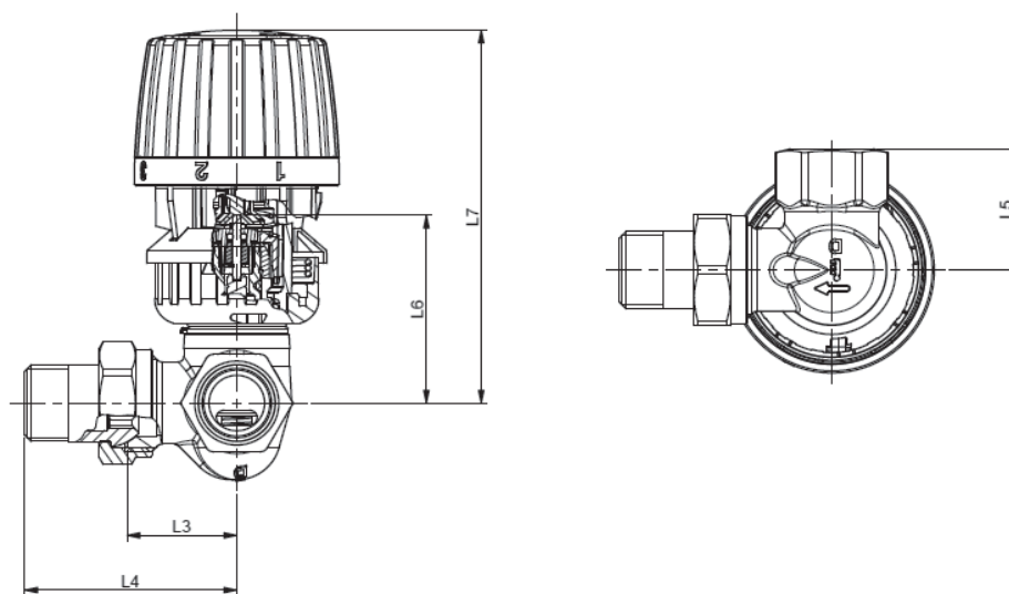
Кутовий клапан RA-DV для монтажу з лівого/правого боку радіатора з термостатичним елементом RA 2991
