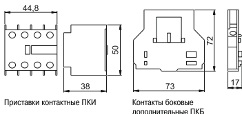
Рисунок 2 – Габаритные размеры приставок
