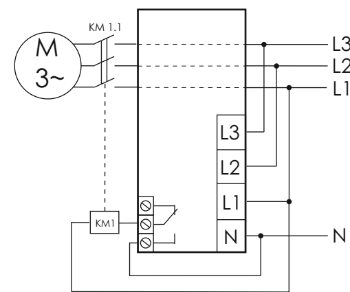
Рис.2 Типовая схема включения изделия AZD для защиты двигателей с рабочим током до 5А.
