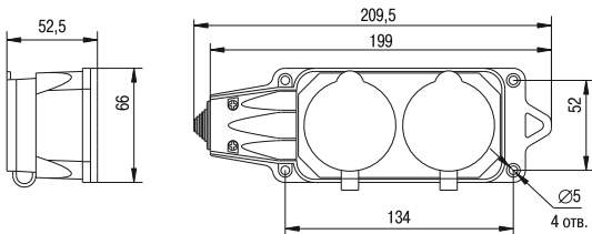
Рисунок 10 – Розетка (колодка) двухместная с защитными крышками РБ32-1-0м
