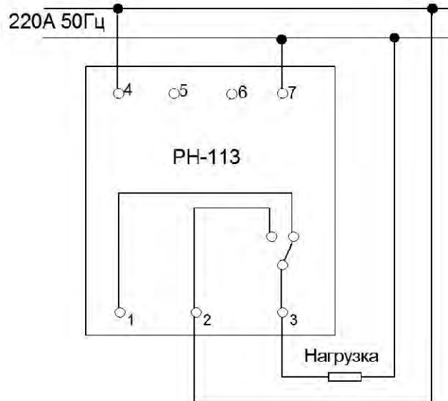
Рисунок 2 – Схема подключения реле
