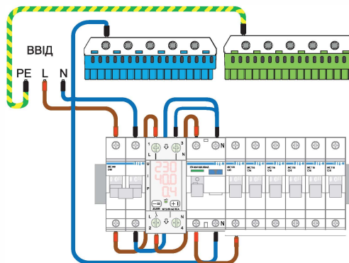
Схема 4. Варіант монтажно-ї схеми без транзиту нуля через ZUBR MF2
