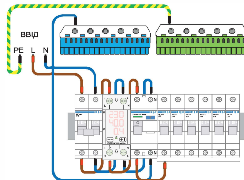
Схема 2. Варіант монтажно-ї схеми з транзитом нуля через ZUBR MF2
