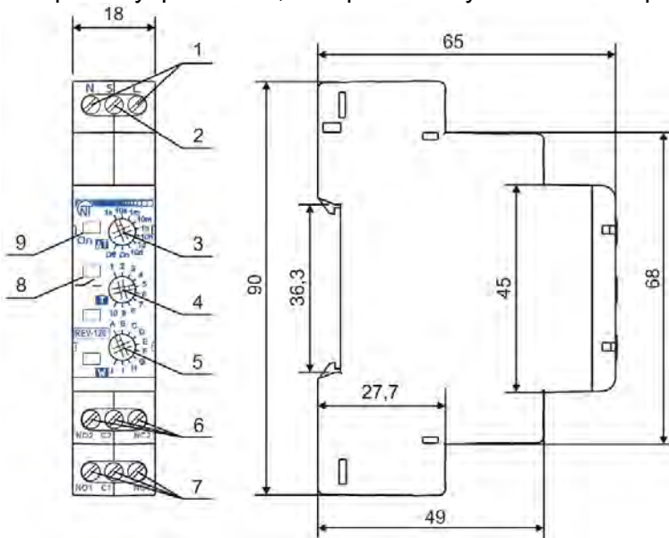
Рисунок 1 – Органы управления, габаритные и установочные размеры REV-120
