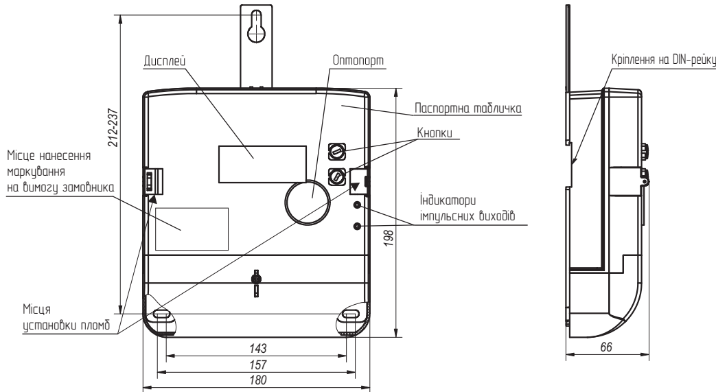
Малюнок А.1 - Загальний вигляд, габаритні і установчі розміри, місця установки пломб на корпусі трифазного лічильника трансформаторного включення типу МТХ 3Г20...D.3...3...4
