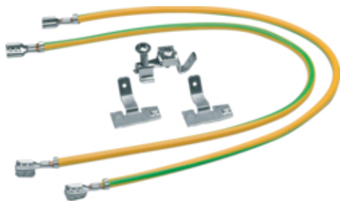
Комплект для заземлення для колон DA 200
