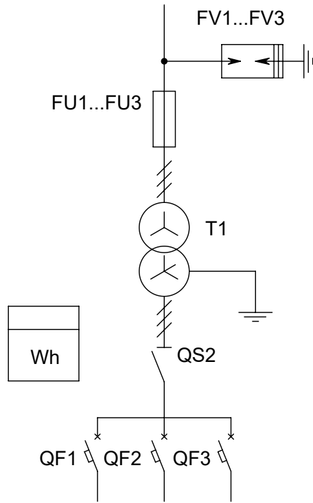
Однолинейная схема КТП1-63 (воздушный ввод)
