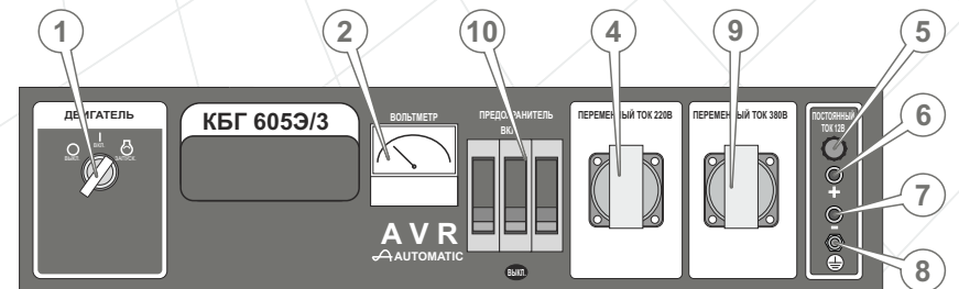
Панель управления КБГ-605Э/3
