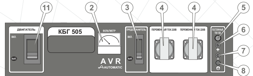
Панель управління КБГ-505
