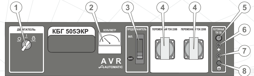
Панель управления КБГ-505ЭКР
