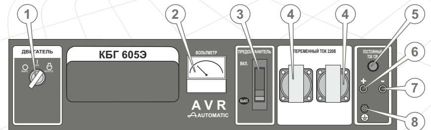
Панель управління КБГ-605Э
