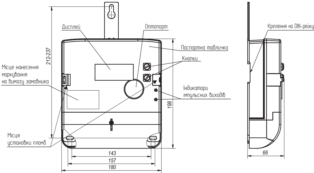
Малюнок А.1 - Загальний вигляд, габаритні і установчі розміри, місця установки пломб на корпусі трифазного лічильника прямого включення типу MTX 3...0.D...4
