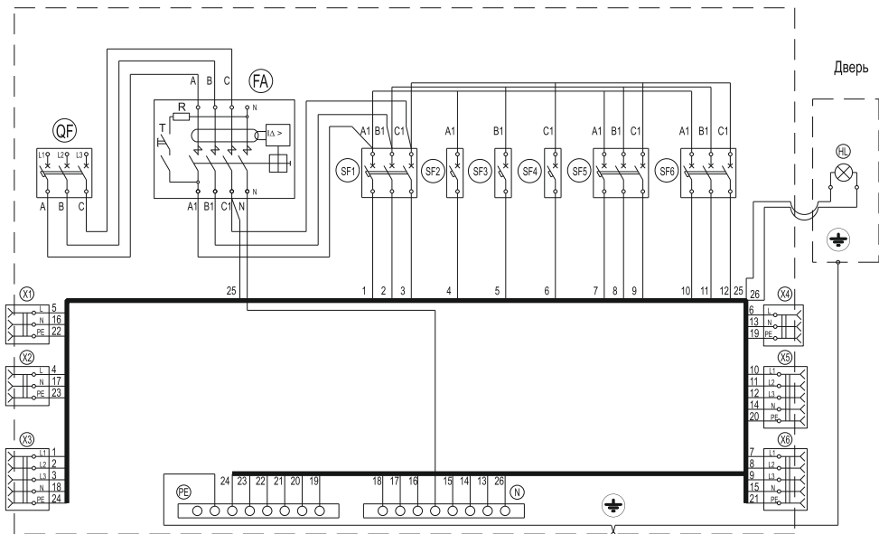
Рисунок 1 – Схема электрическая
