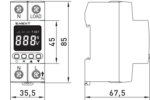
Рис. 1 Габаритні розміри
