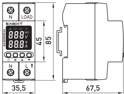
Рис. 1 Габаритні розміри
