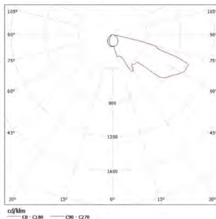
KANLUX S.A. (kat 4680) DORA LED-J01 / Krzywa rozsyłu światła (biegunowo)
