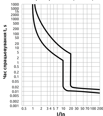
Характеристика D (63-125A)
