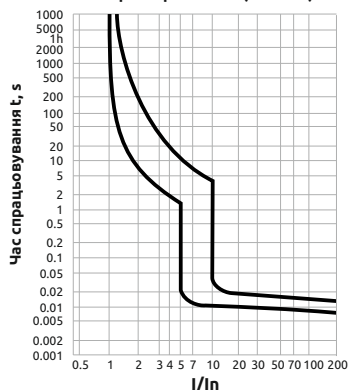
Характеристика C (63-125A)
