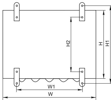
Рисунок 1 – Вид корпуса сзади
