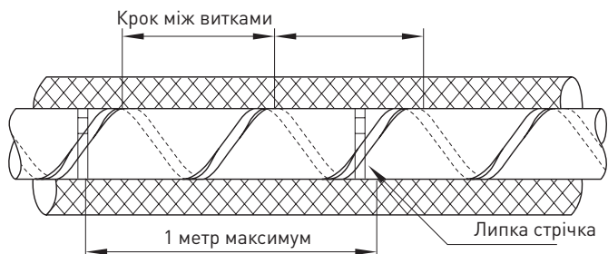
Суцільне кріплення
