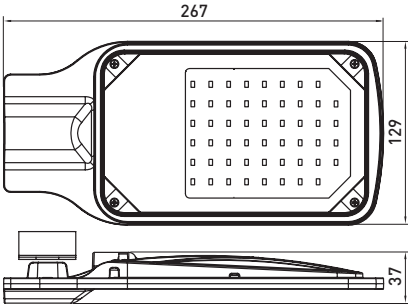
Рис. 1 e.LED.street.stand.30.6500
