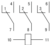
Рисунок 2. Схемы электрические принципиальные
