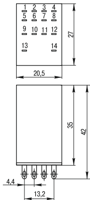
Рисунок 1. Габаритные размеры
