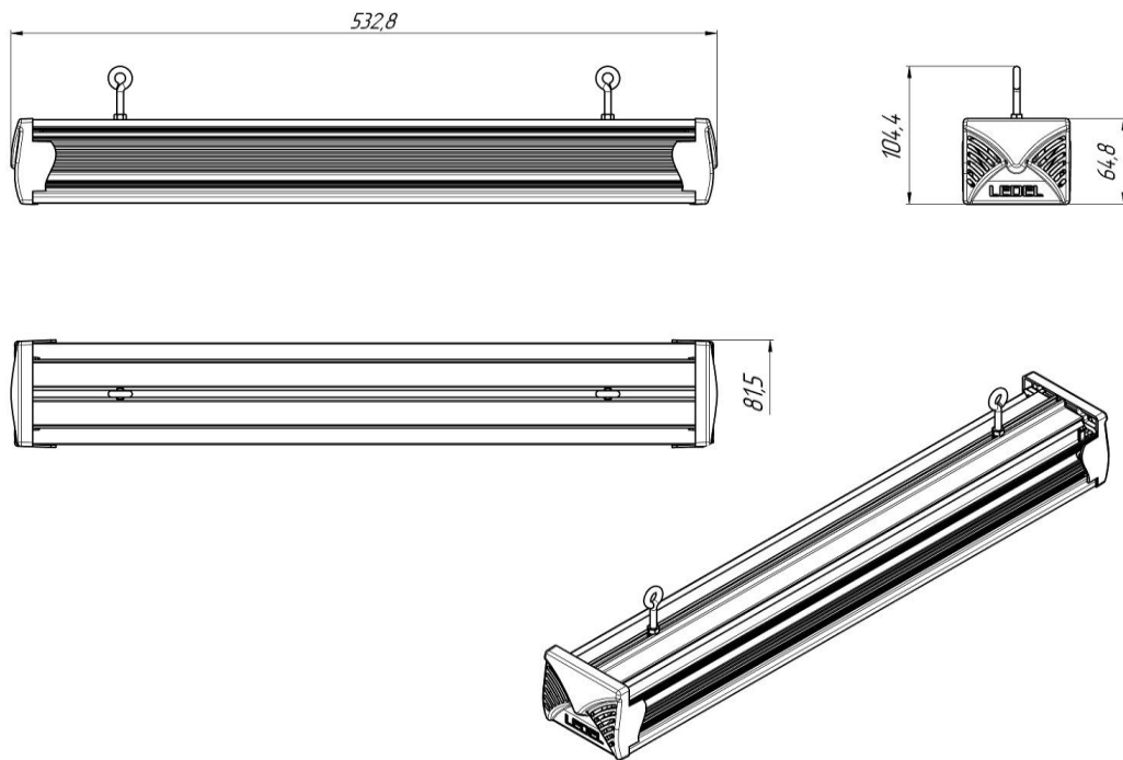
Рисунок 2 Светильник «L-industry NEW 24». Подвесной вариант
