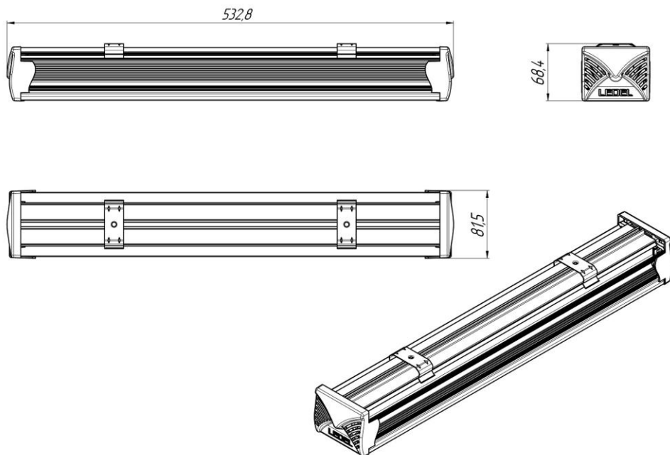
Рисунок 3 Светильник «L-industry NEW 24». Задвижной вариант
