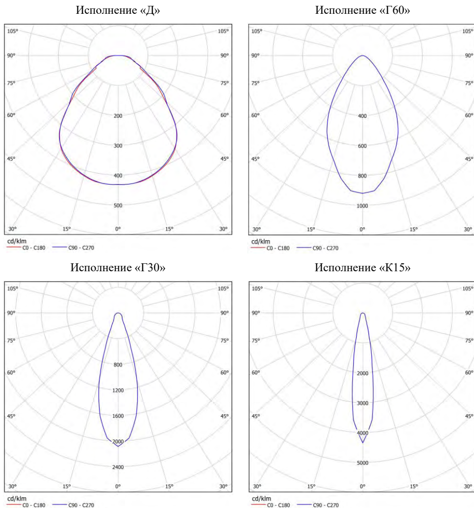
Рисунок 7 Тип КСС
