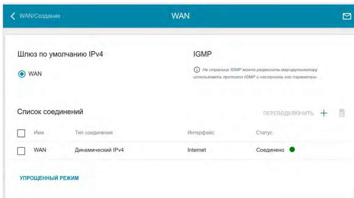
Рисунок 53. Страница Настройка соединений / WAN . Расширенный режим.
