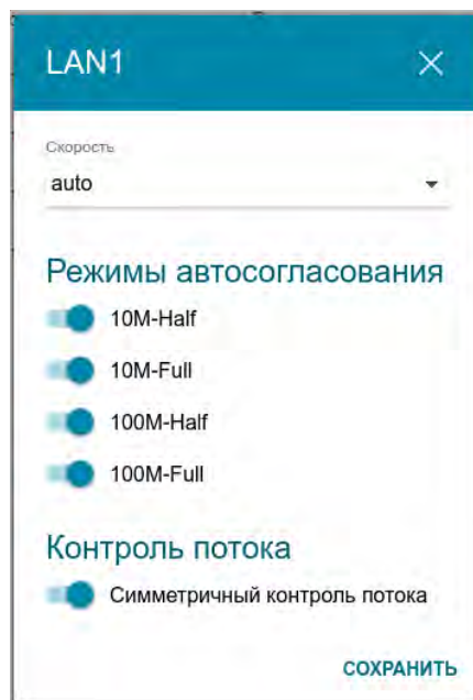
Рисунок 105. Окно изменения настроек порта маршрутизатора.
