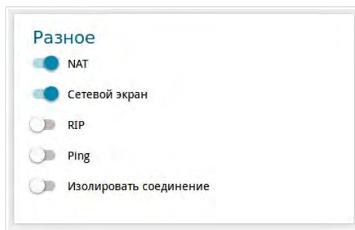
Рисунок 68. Страница добавления соединения типа PPTP . Раздел Разное .
