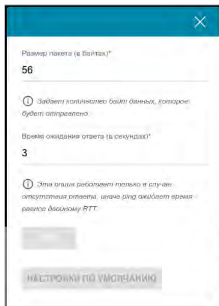
Рисунок 133. Страница Система / Пинг . Окно дополнительных настроек.
