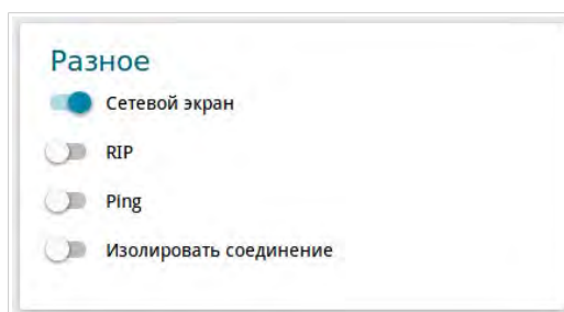
Рисунок 73. Страница добавления соединения типа PPPoE IPv6 . Раздел Разное .
