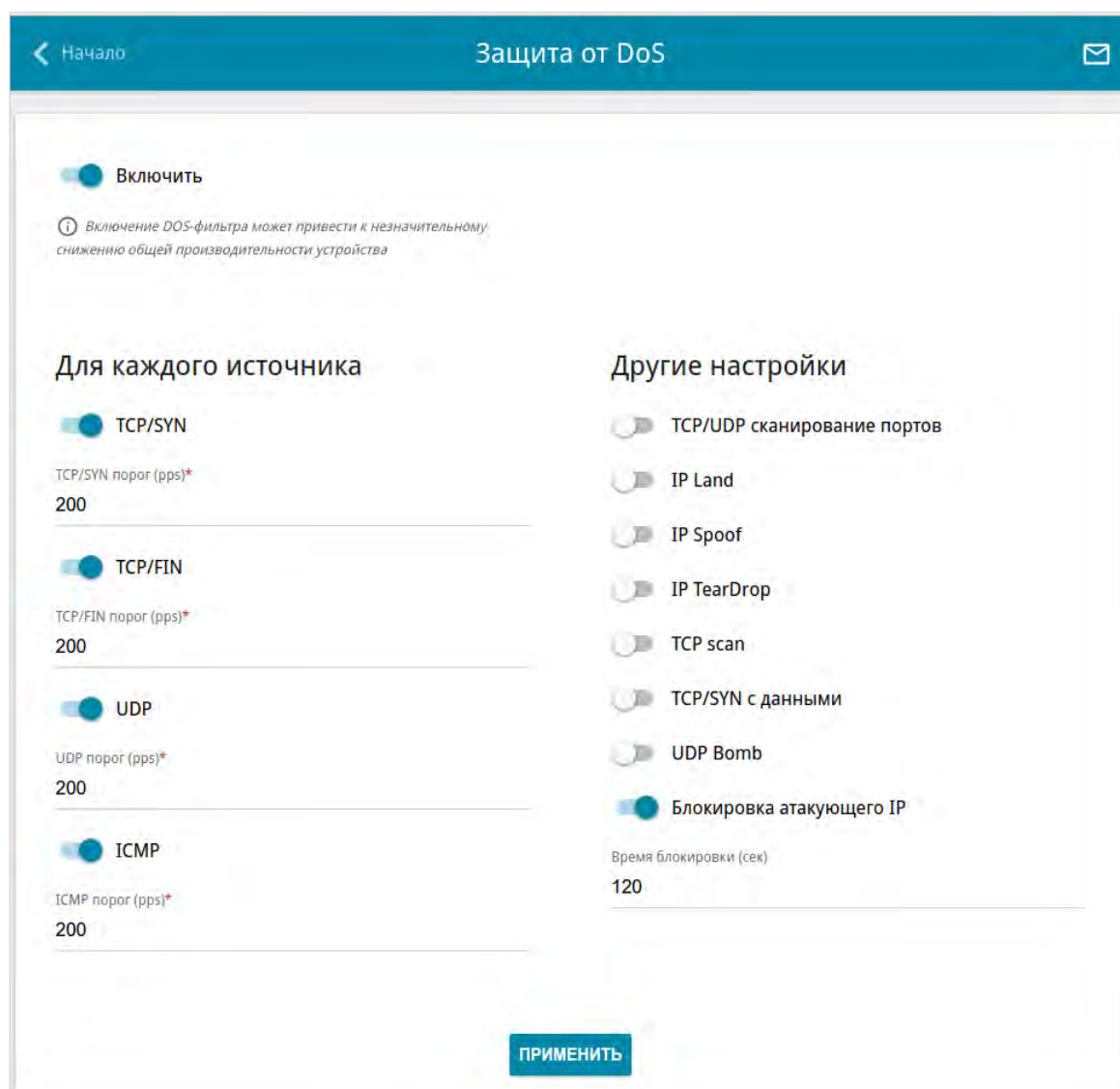
Рисунок 127. Страница Межсетевой экран / Защита от DoS .
