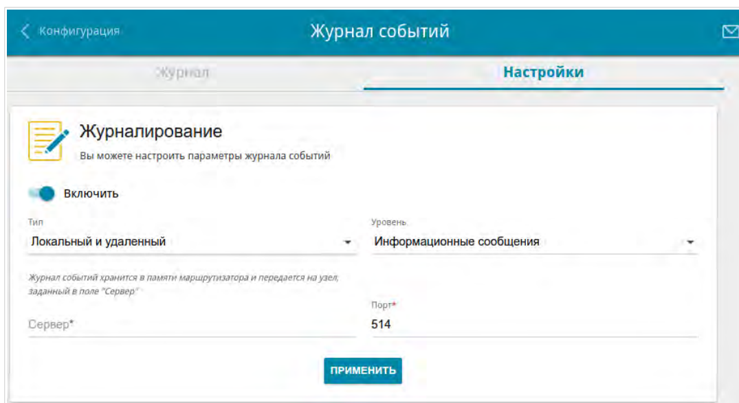
Рисунок 130. Страница Система / Журнал событий . Вкладка Настройки .
