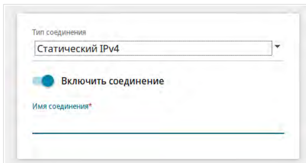
Рисунок 54. Страница добавления соединения типа Статический IPv4 . Выбор типа соединения.
