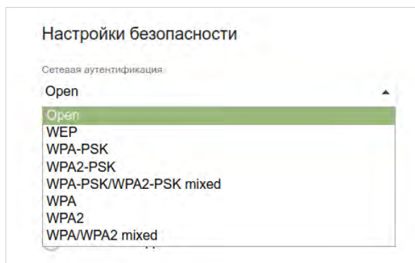
Рисунок 83. Типы аутентификации, поддерживаемые маршрутизатором.
