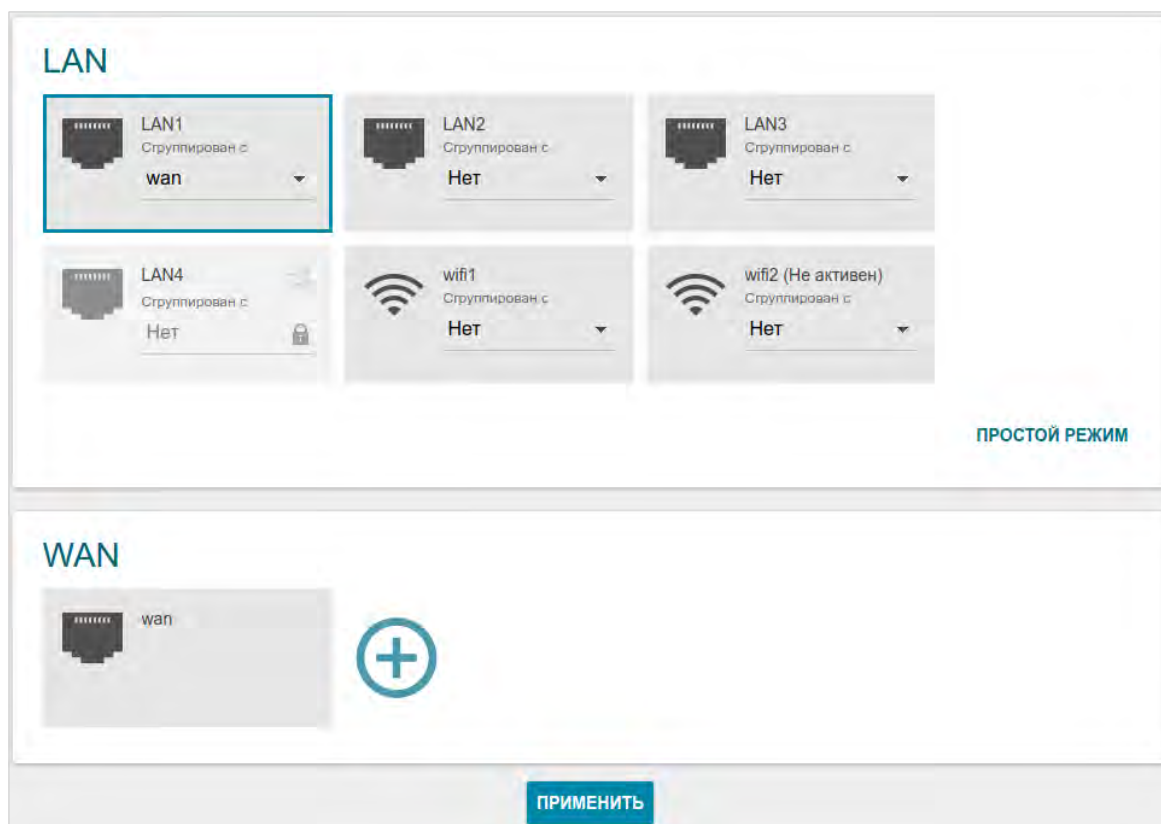
Рисунок 43. Мастер подключения мультимедиа-устройств. Расширенный режим.
