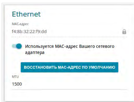
Рисунок 70. Страница добавления соединения типа PPPoE IPv6 . Раздел Ethernet .
