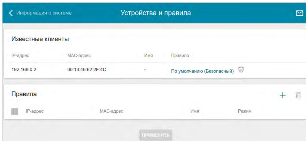
Рисунок 139. Страница Яндекс.DNS / Устройства и правила .
