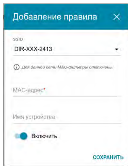
Рисунок 96. Окно для добавления правила MAC-фильтра.
