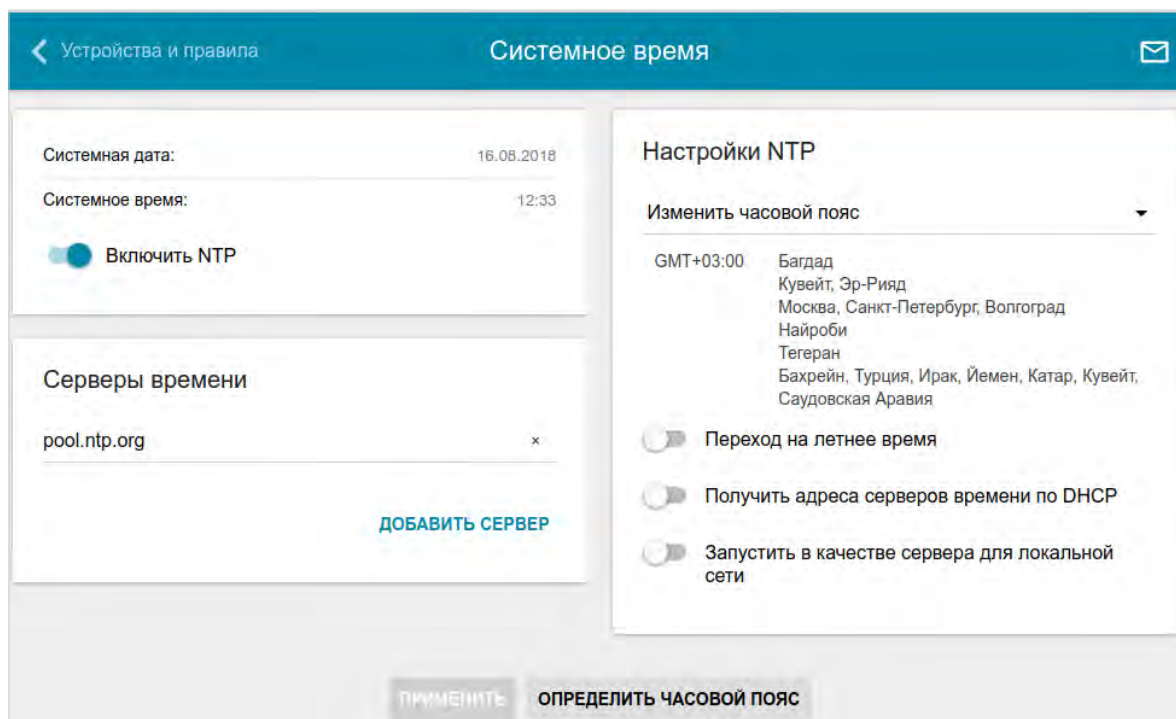
Рисунок 137. Страница Система / Системное время .
