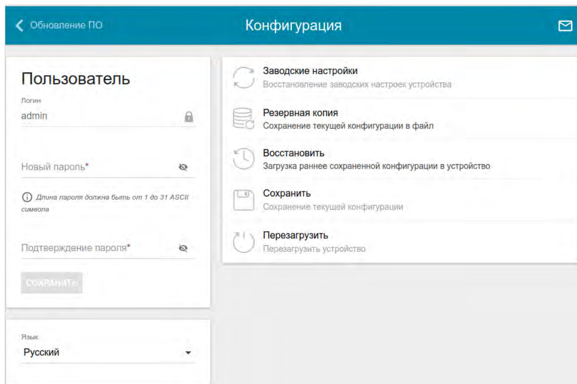
Рисунок 128. Страница Система / Конфигурация .
