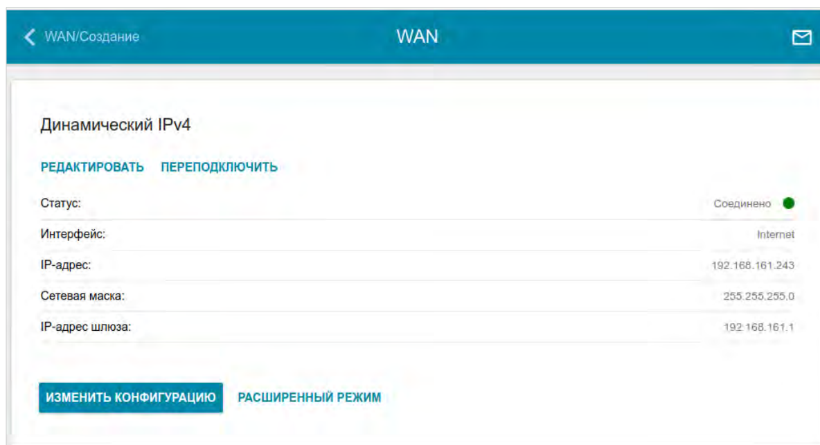
Рисунок 52. Страница Настройка соединений / WAN . Упрощенный режим.
