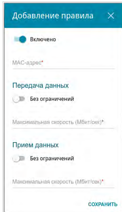
Рисунок 93. Окно для настройки ограничения скорости.
