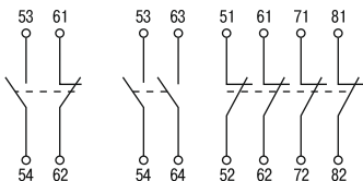
Рисунок 3. Электрические схемы ПКИ
