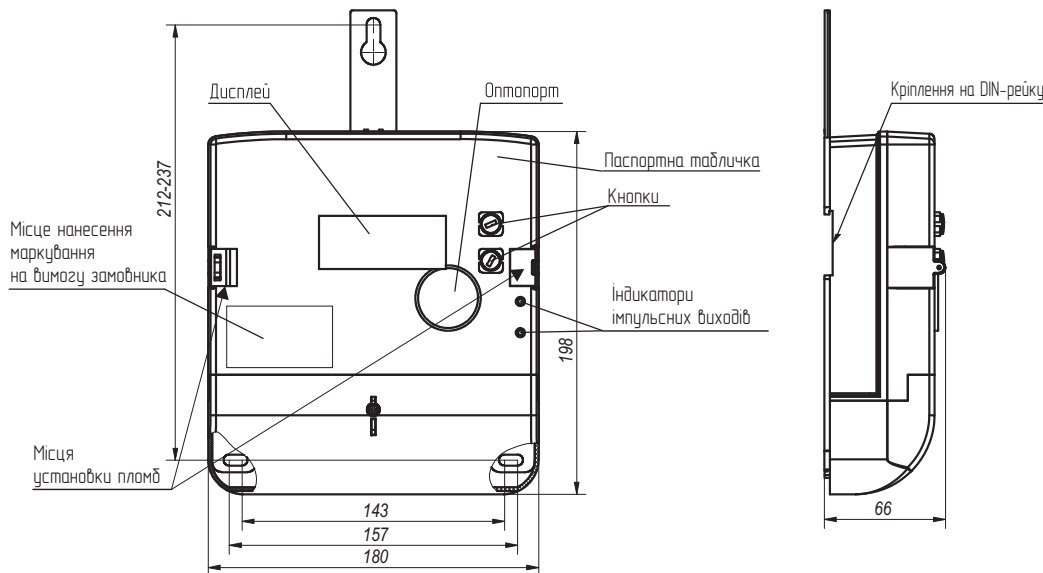
Малюнок А.1 - Загальний вигляд, габаритні і установчі розміри, місця установки пломб на корпусі трифазного лічильника трансформаторного включення типу MTX 3G20...D.3...3...4
