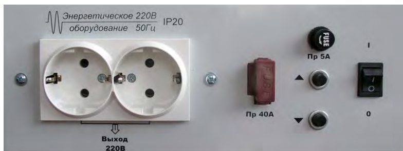
Рис.4.Верхняя панель.
