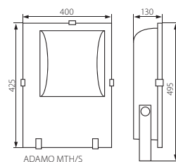
ADAMO MTH/S
