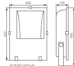
ADAMO MTH/A
