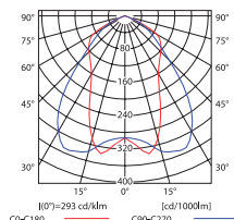
ADAMO MTH-400/S
