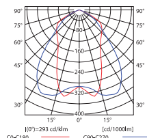
ADAMO MTH-250/S
