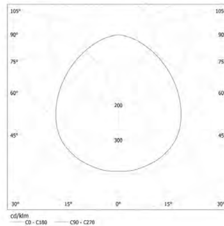
KANLUX S.A. (kat 22190) PAX TL-90LED / Krzywa rozsyłu światła (biegunowo)
