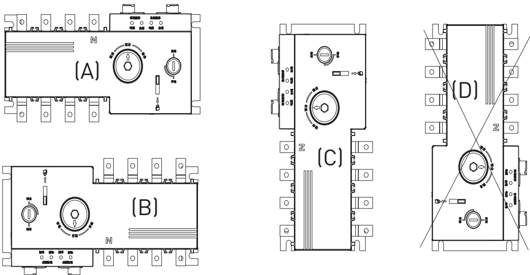
Рис. 4 Варіанти монтажу ABP (A, B, C – правильно, D – неправильно)
