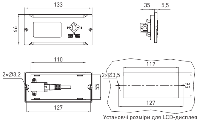
Рис. 6 Габаритні та установчі розміри LCD-дисплея (мм)
