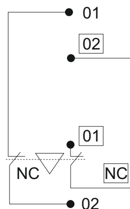
Принципова схема
