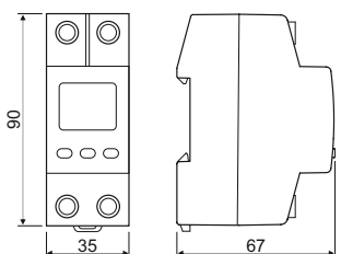
Габаритні розміри
