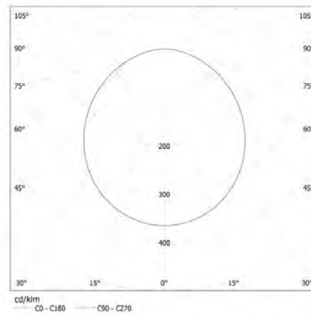
KANLUX S.A. (kat 25825) KATRO N LED 24W-WW / Krzywa rozsyłu światła (biegunowo)
