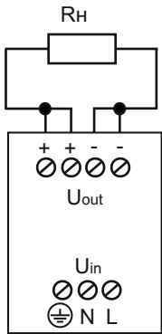
Rn - нагрузка подключаемая к блоку питания
