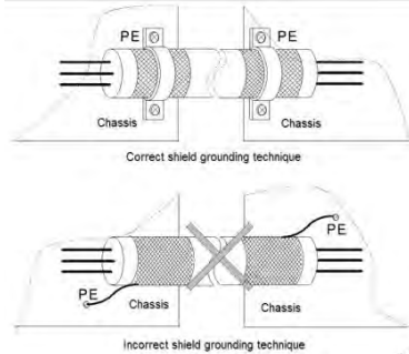
Рис 4-18. Техника заземления 360 градусов
