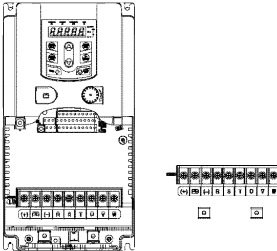
Рис. 4-10. 7.5~15 кВт клеммы силовых цепей
