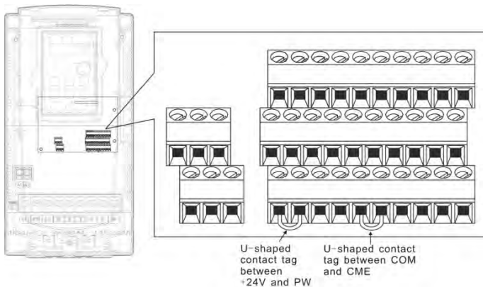
Рис. 4-21. U-образный контакт
