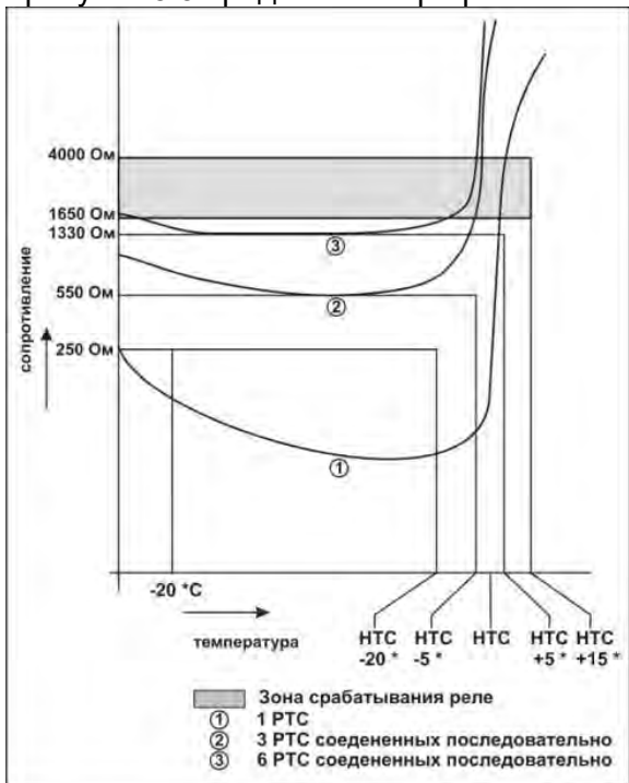
Рисунок 5.3 – График зависимости сопротивления датчика PTC от температуры
