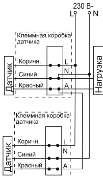
Рисунок 19 – Схема параллельного подключения датчиков
