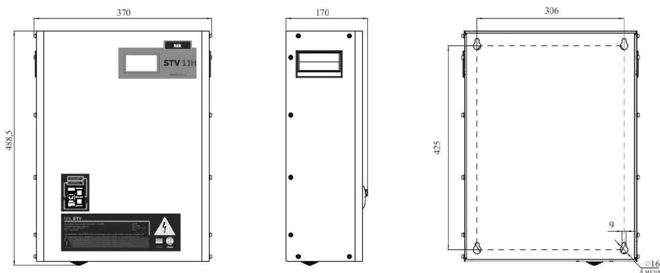
Рис.3.1 Габаритні та установочні розміри стабілізаторів STV-11H
