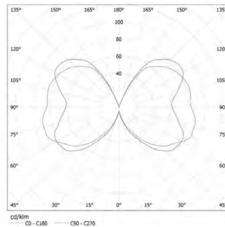
KANLUX S.A. (kat 26041) ST64 FILLED 6W E27-WW / Krzywa rozsyłu światła (biegunowo)
